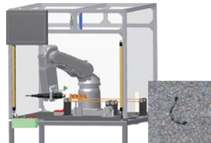
ロボットに取り付けたカメラで樹脂部品の表面を撮像し、画像処理検査を行う
