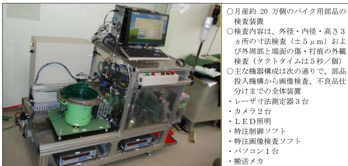
図表 3.5 外観検査（画像処理）装置の例
